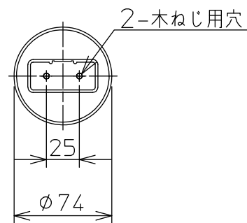
取付部詳細
