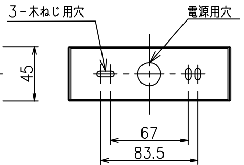
取付部
