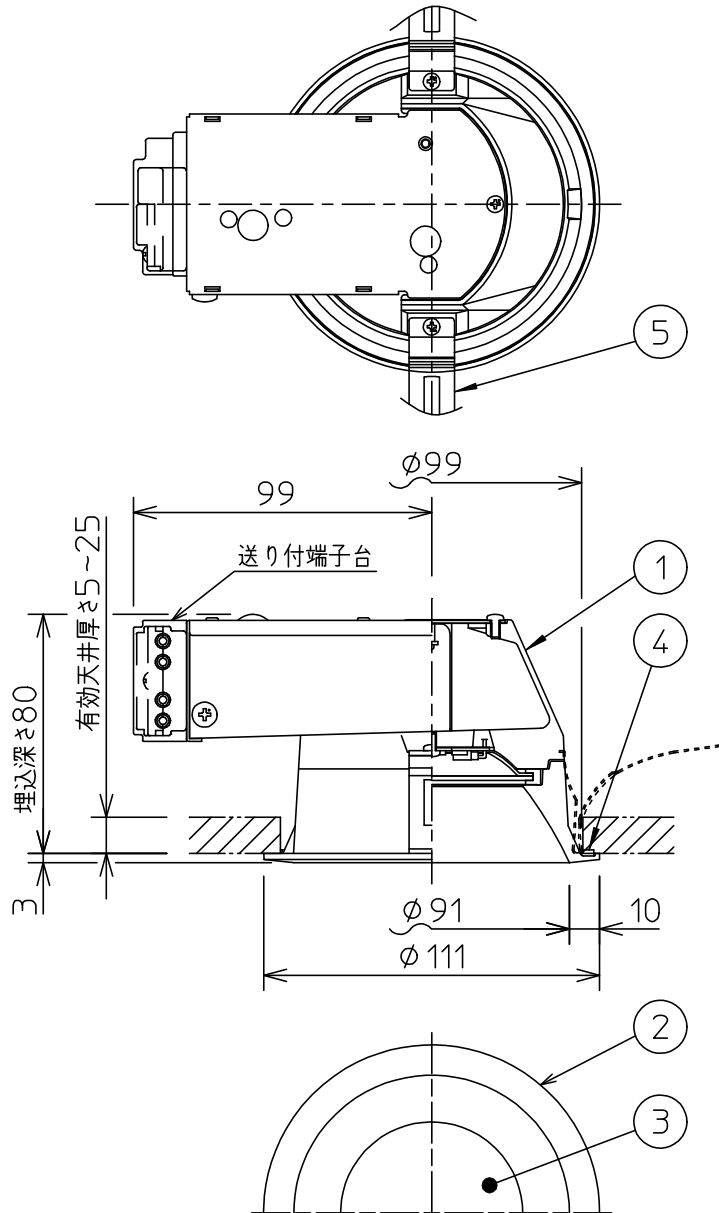
埋込穴寸法
